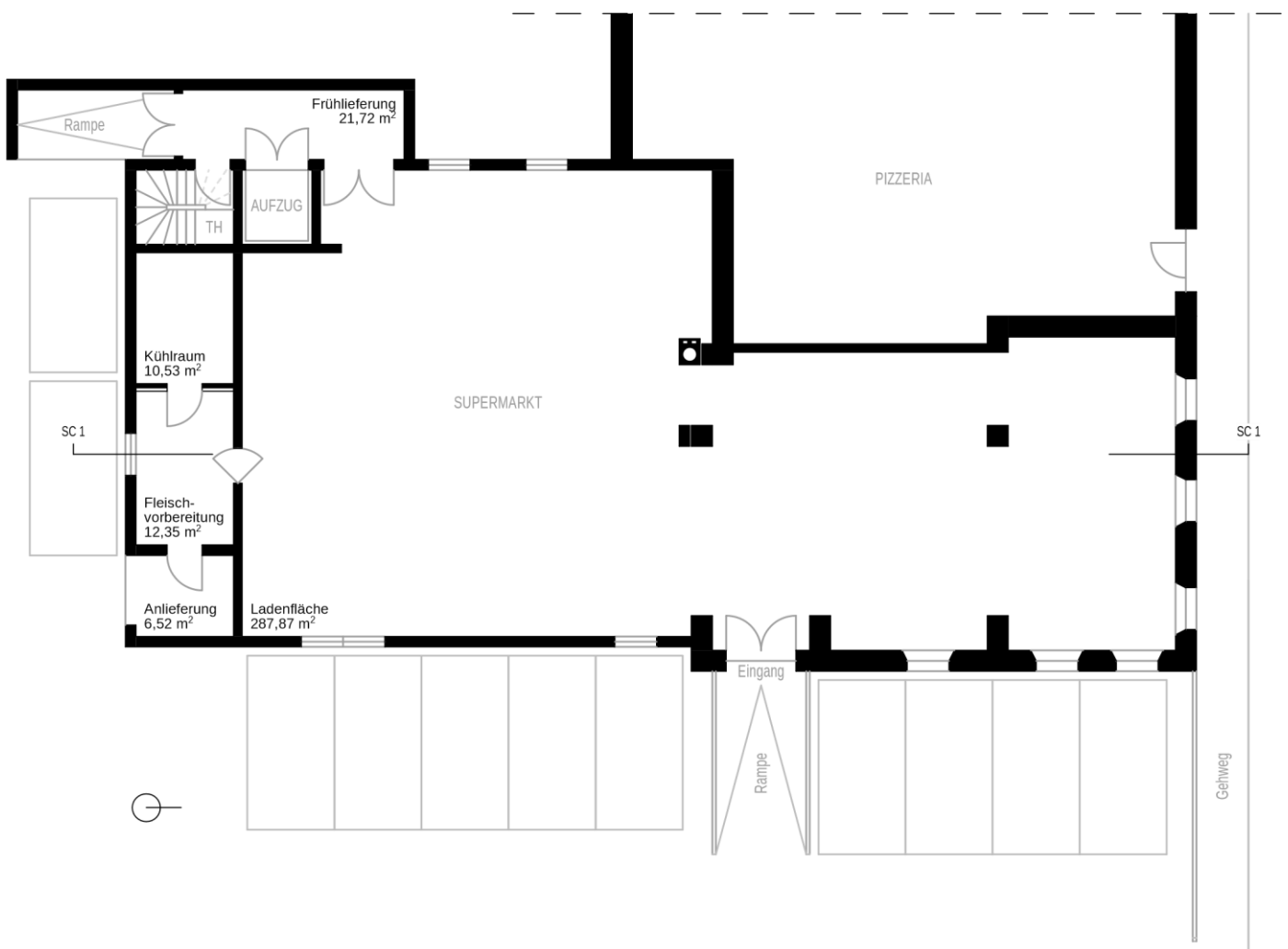
GRUNDRISS EG M 1 : 100
